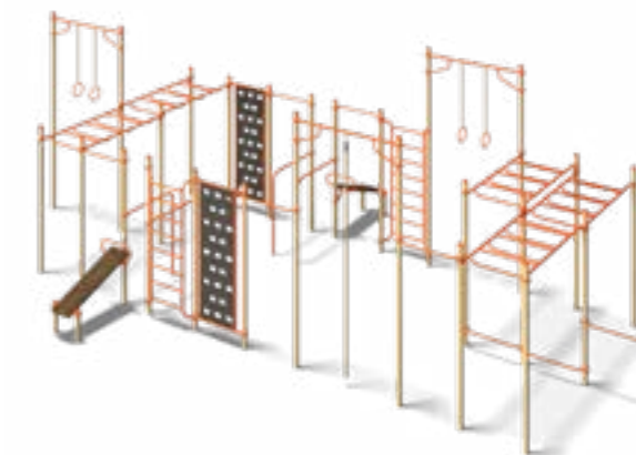
ЛГВО-30 Спортивный комплекс
