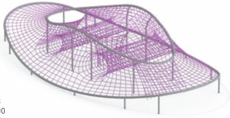
ЛГСК-11.7106 Канатный комплекс «Одиссей»
